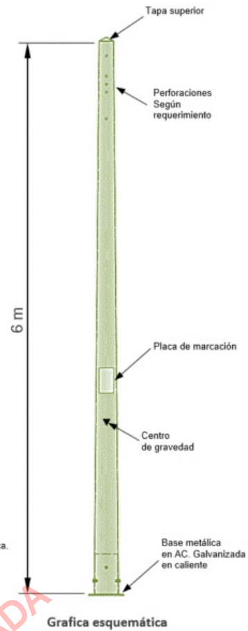
Grafica esquemática
