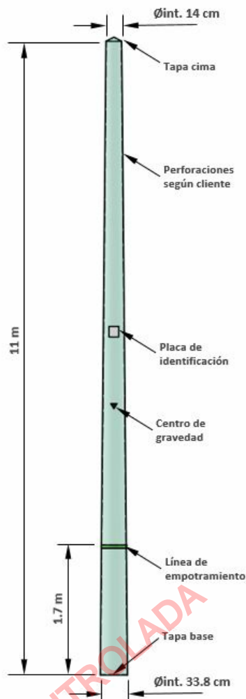
Grafica esquemática
